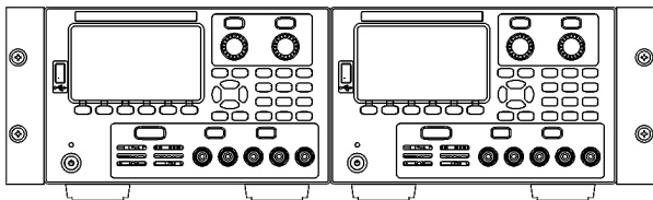
핸들이 없는 랙 장착 키트(1CM104A)
